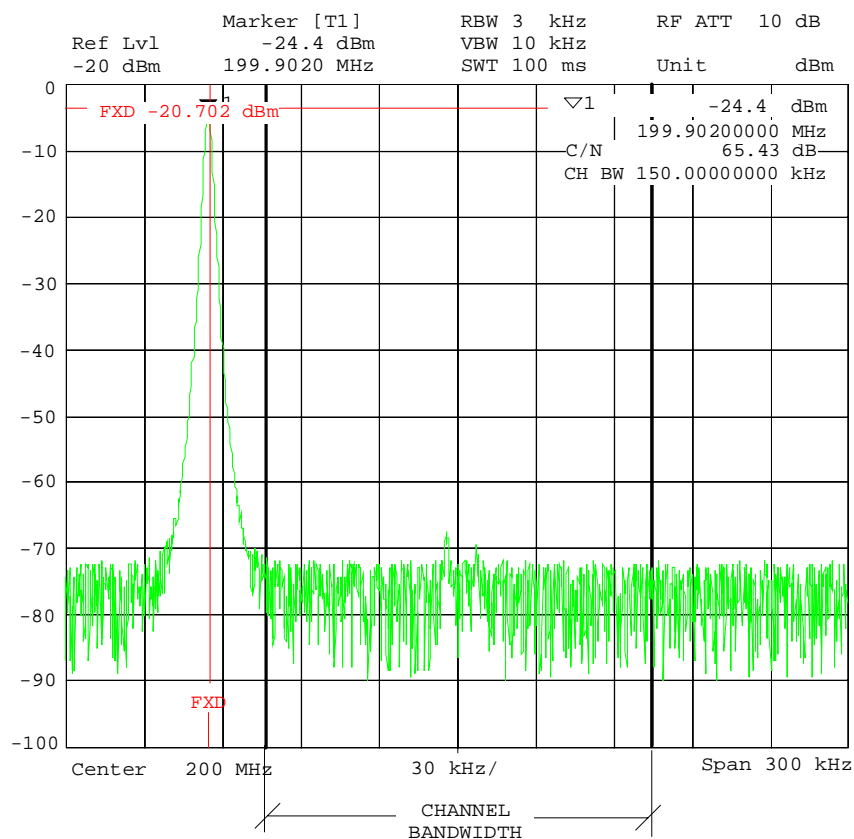
Bild 4-5 Meßbeispiel: Messung der Signal-/Rauschleistung
