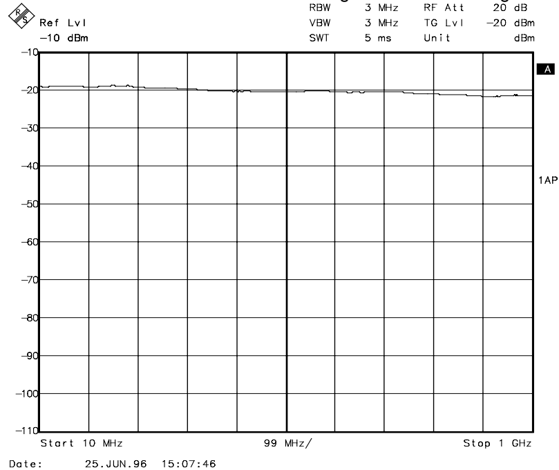
Bild 4-16 Meßkurve des Kalibriervorgangs einer Transmissionsmessung
